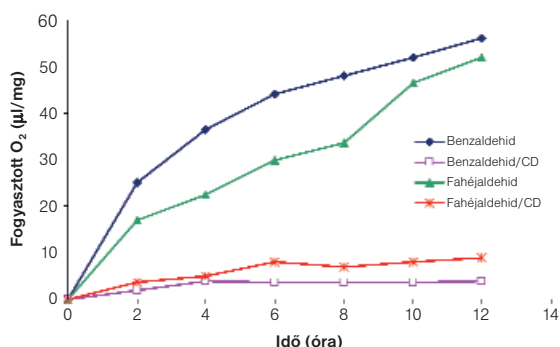
4. ábra. A szabad és a komplexbe zárt benzaldehid és a fahéjaldehyde oxigénfogyasztása Warburg-készüléken meghatározva
