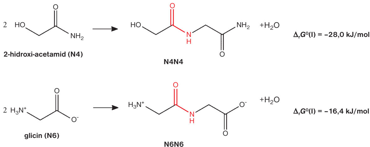
3. ábra. A polikondenzációs reakciók első lépései és a hozzájuk tartozó reakció-szabadentalpiák ( \Delta_r G^\circ(\text{I}) ). Pirossal jelöltük a molekulák peptidkötését
