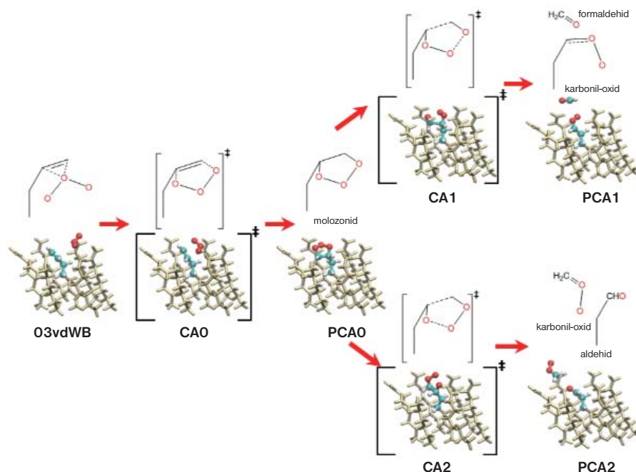
5. ábra. A szerves felület ózonos oxidációjának (ózonolízis) mechanizmusa és az elemi lépésekhez tartozó számított térszerkezetek. Az átmeneti állapotokhoz tartozó szerkezeteket zárójellel és ‡ szimbómmal jelöltük
