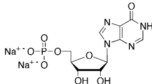
11. ábra. Dinátrium-inozinát [27]
