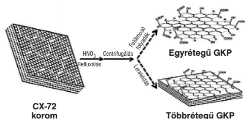
7. ábra. Egy- és többretegű GKP-k előállítása oxidálással [16]
