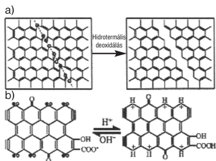
6. ábra. „Lentről felfelé” hidrotermális módszer GKP-k előállítására [15]
