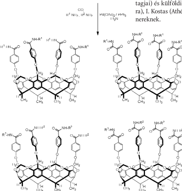
8. ábra. Tetrajód-kavitand palládium katalizált aminoszterán karbonilezése
