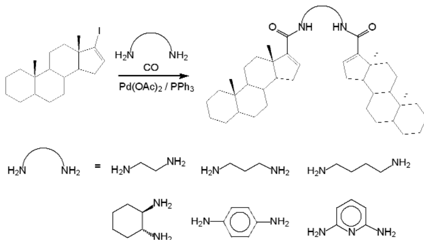
7. ábra. Szteránvázis jódarkének aminokarbonilezése diaminok mint nukleofilek jelenlétében
