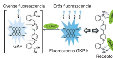
20. ábra. Glükóz kimutatása bipiridinium-sóval kezelt GPK-kel
