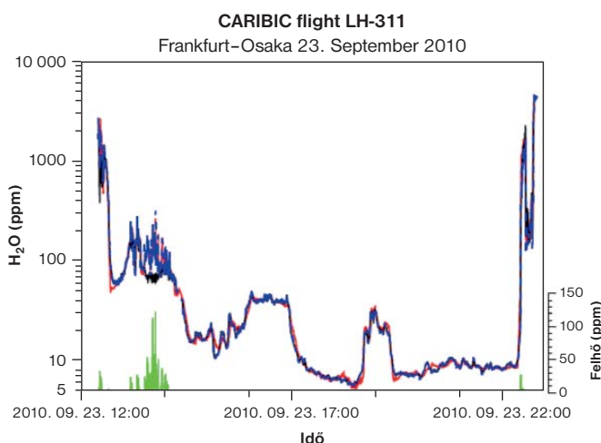
5. ábra. Atmoszférikus vízgőz (fekete görbe) és a teljes víztartalom (piros görbe: fotoakusztikusan mért, kék görbe: referencia-módszerrel mért), valamint a kettő különbségéből számolt felhőcsepp-koncentráció (zöld görbe) mérése fotoakusztikus rendszerrel egy repülőgépes út során
