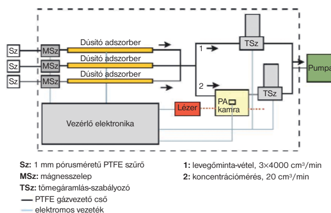
7. ábra. Három különböző mérési magasságban nagy pontossággú ammóniakoncentráció-mérésre alkalmas fotoakusztikus berendezés
