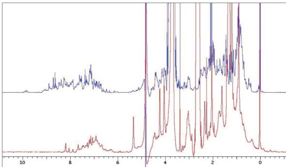
1. ábra. Egy közepes méretű (17 kDa) rekombináns fehérjét tartalmazó készítmény (felül), valamint egy közel hétszer több ^1\text{H} -atommal rendelkező monoklonális antitestet (150 kDa) tartalmazó készítmény 1D ^1\text{H} NMR-spektruma (alul). Utóbbi a molekula méretéből adódó zsúfoltság és jelszélesedés miatt jóval kevesebb értékelhető jelet tartalmaz
