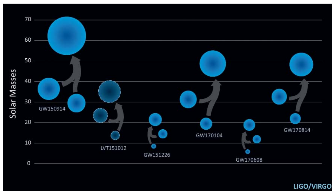
Ismert tömegű fekete lyukak
