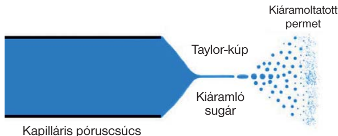
3. ábra. A Taylor-kúp következtében kialakuló ionos folyadék-permet kíáramoltatása
