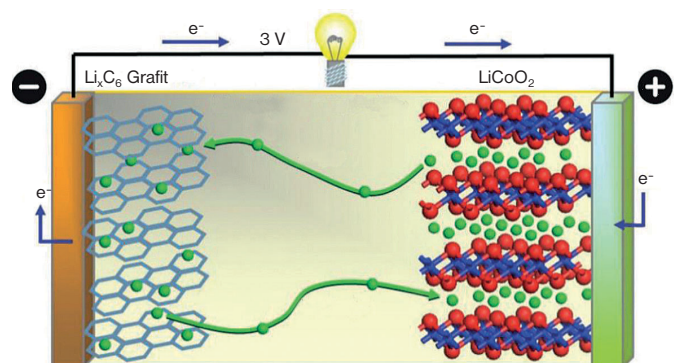
2. ábra. A zöld gömbbel jelzett Li-ionok töltéskor a szénelapú, kisütéskor pedig a fém-oxid-elektrodhoz vándorolnak [3]
